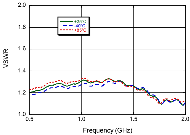
VSWR
