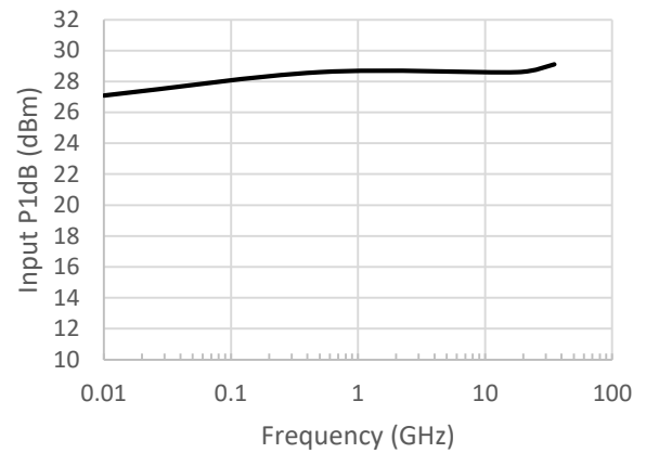
Input P1dB
